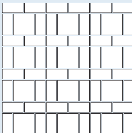
Макет H5 - 318x318 мм
